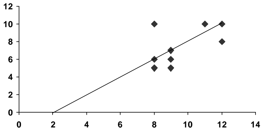
Рис. 7. Линия регрессии.
