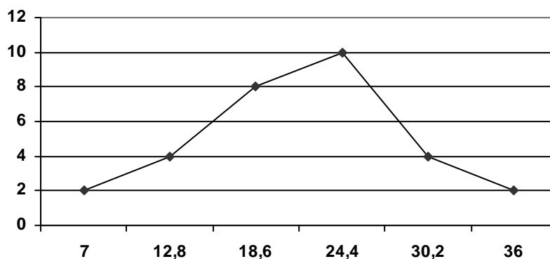
Рис.2. Полигон распределения.
